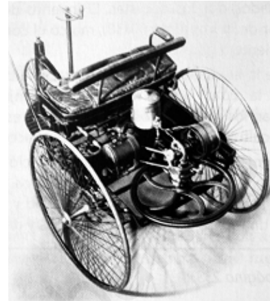
Fig 16: Autocarro de tres ruedas de un único cilindro y 0.9 CV capaz de alcanzar los 16 km/h construido por Karl Benz (Benz Motocarro patentado 1)
