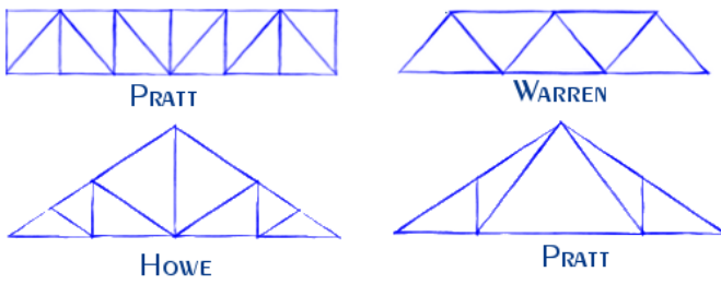
Fig 11: Algunos tipos de cerchas
