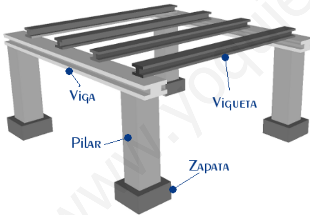
Fig 6: Zapata, pilar, viga y vigueta.
