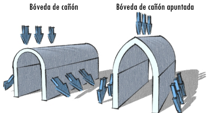
Fig 16 Cargas y tensiones en una bóveda. Puede verse que el empuje lateral es mucho menor en el caso de la bóveda apuntada.
