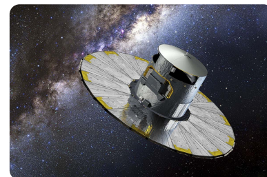
Misión Gaia (astrometría de la galaxia) ESA (Agencia Espacial Europea)
