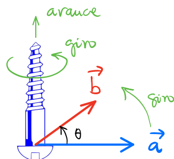
Regla de la mano derecha
