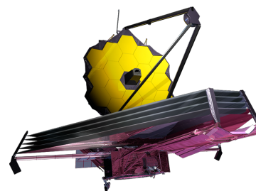
Telescopio espacial James Webb NASA / ESA / CSA
