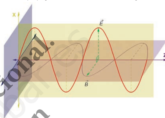
Vibración del campo eléctrico, E , y magnético, B , en la propagación de una onda electromagnética
