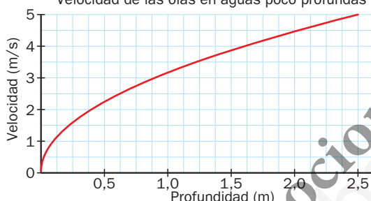
Velocidad de las olas en aguas poco profundas
