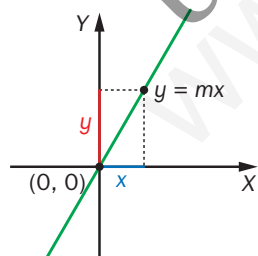
Función lineal
