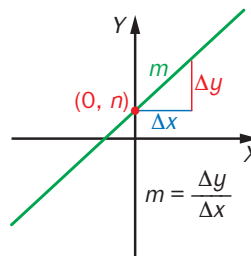
Función afín
