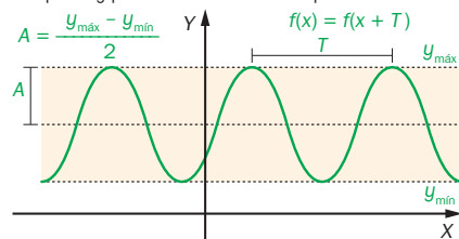
Amplitud y periodo de una función tipo seno o coseno
