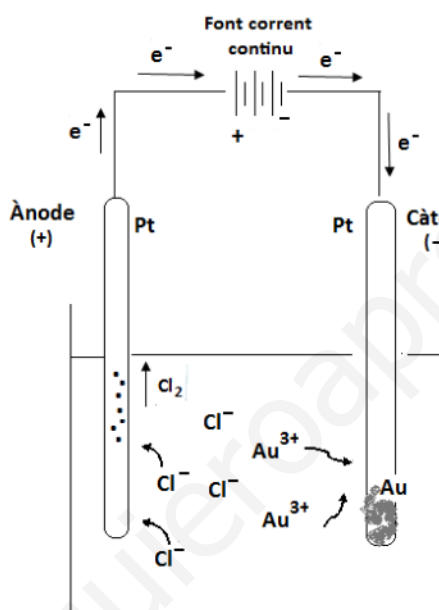
Disolució de \text{AuCl}_3
