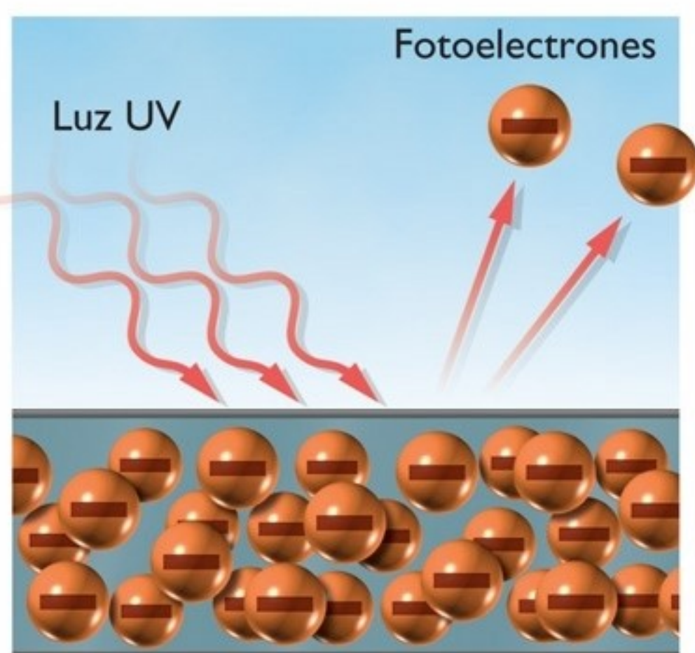
Efecto fotoeléctrico.
