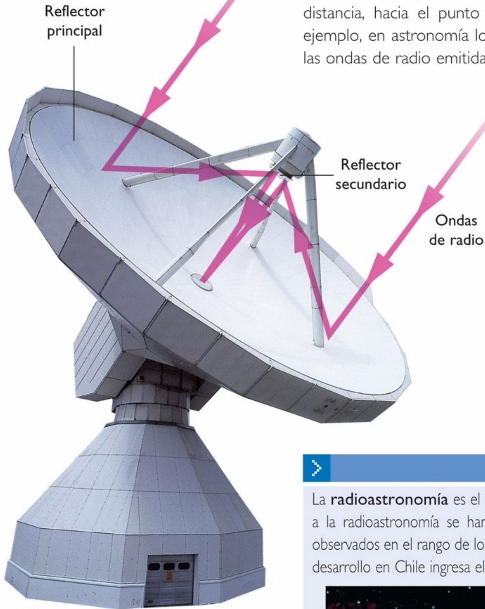
Radiotelescopio.
