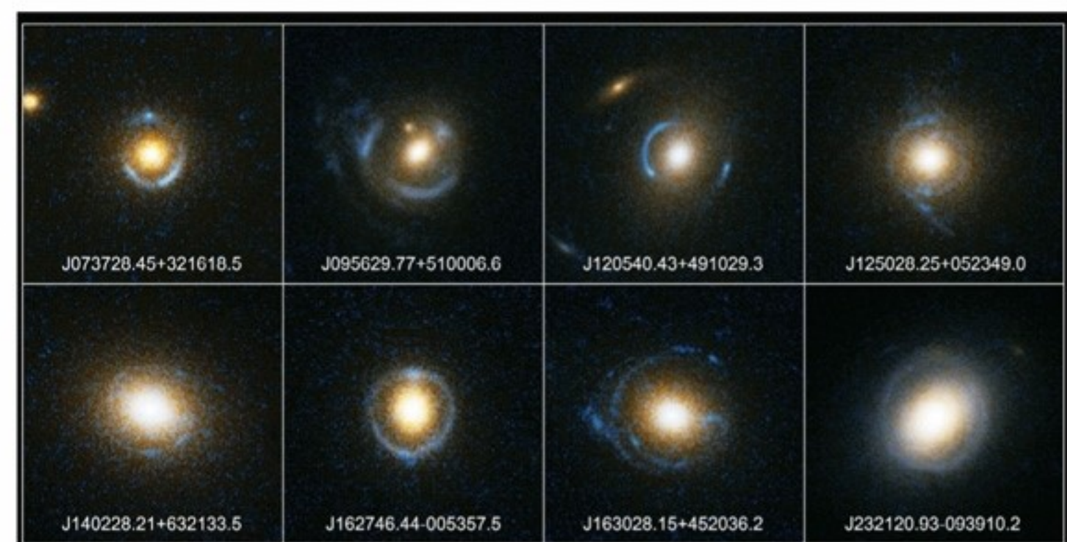
Anillos de Einstein
